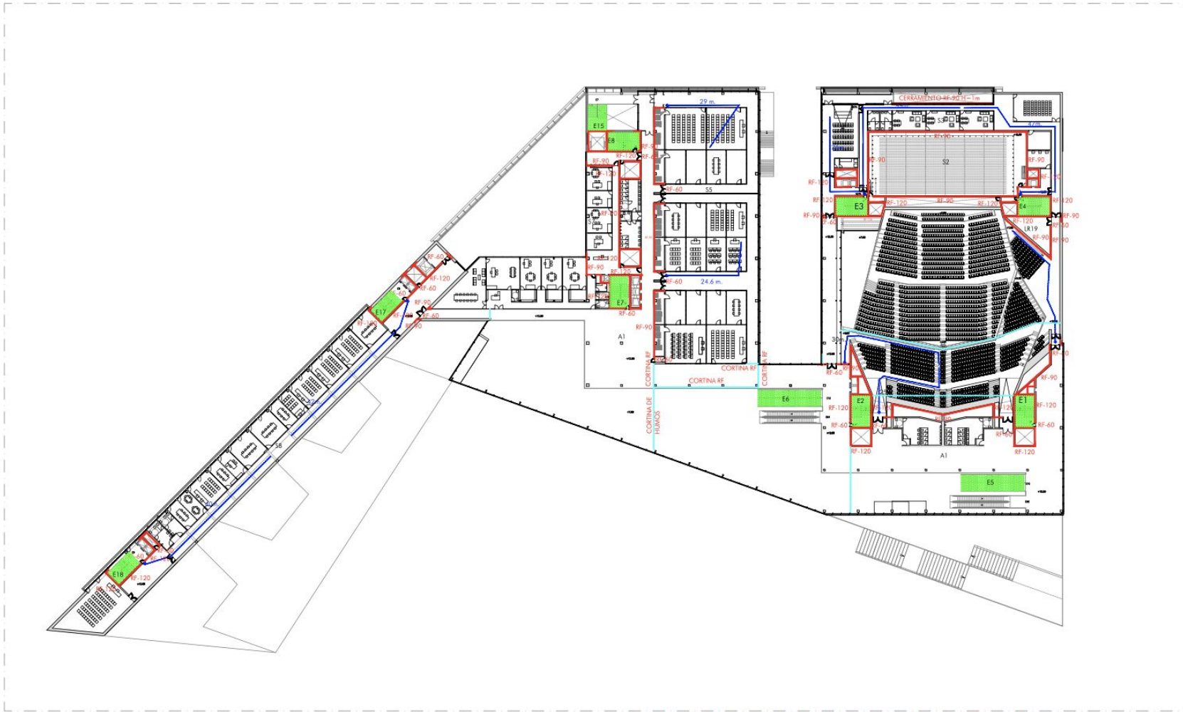
PLANTA COTA +12,50 M
