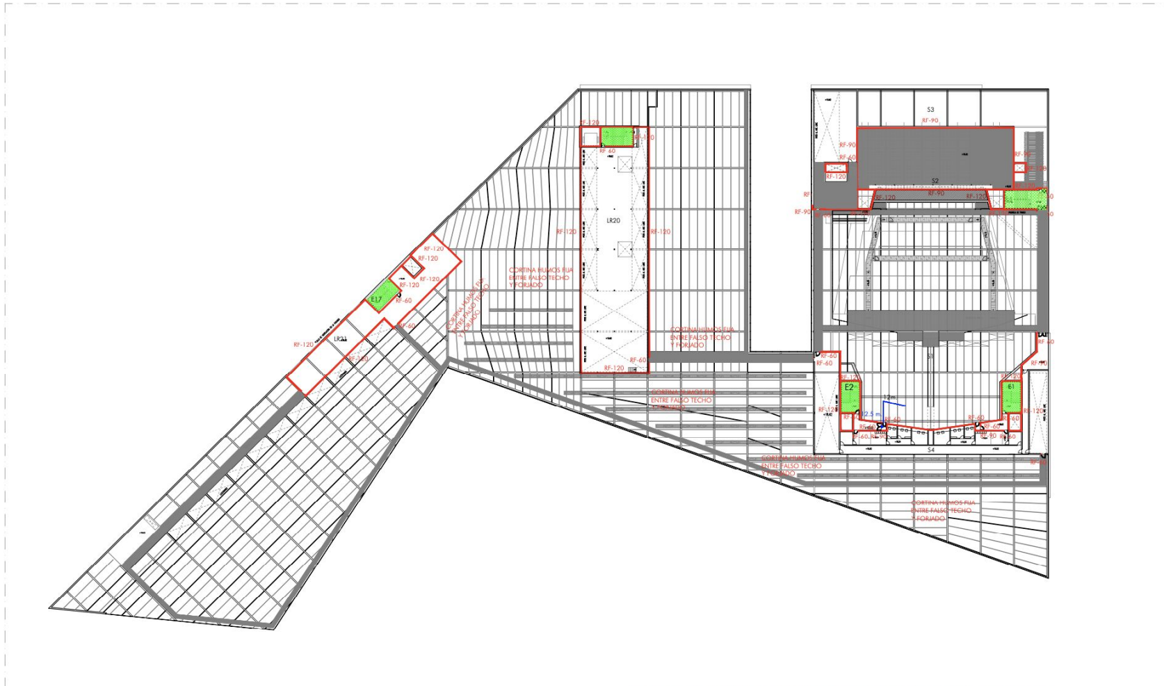
PLANTA COTA +18,62 M
